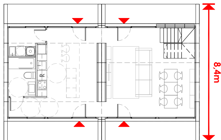
PLANTA BAIXA
