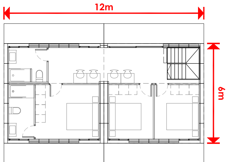
PLANTA PRIMERA
